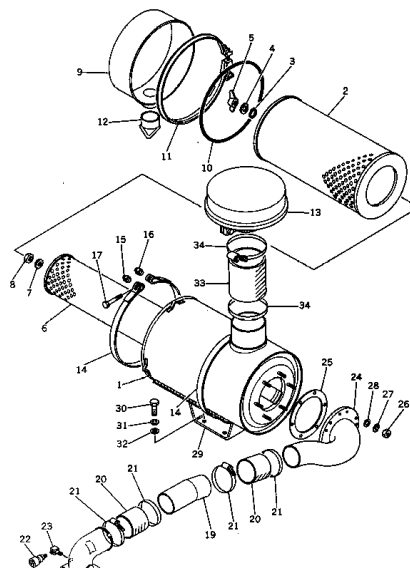
エアー クリーナー FIG. 162 AIR CLEANER
