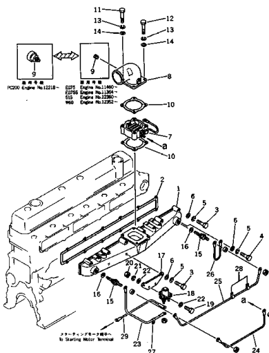
エア インテーク マニホールド および コネクション FIG. 113 AIR INTAKE MANIFOLD AND CONNECTION 適用機 (EG75 ENGINE NO. 11460-17419) (EG75S ENGINE NO. 11364-17419)
