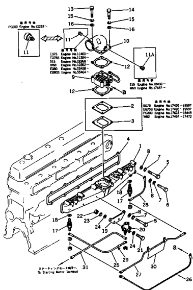
エア インテーク マニホールド および コネクション FIG. 113A AIR INTAKE MANIFOLD AND CONNECTION (EG75 ENGINE NO. 17420- ) (EG76S ENGINE NO. 17420- )
