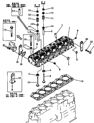
シリンダヘッド FIG. 101 CYLINDER HEAD
