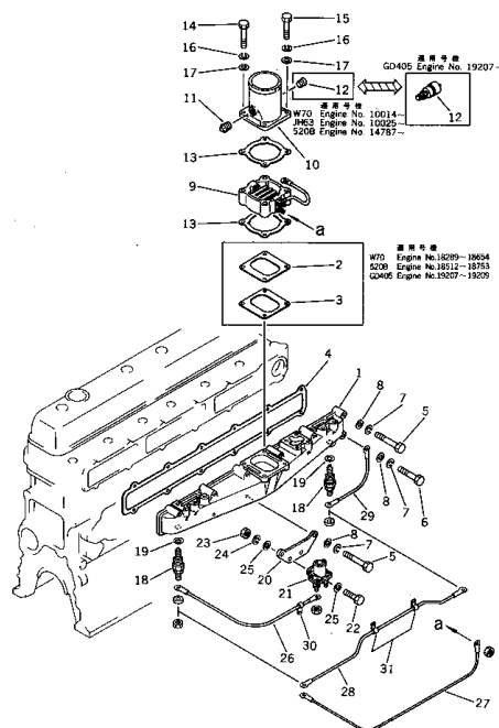
エアインテークマニホールドおよびコネクション 適用号機 FIG. 111A AIR INTAKE MANIFOLD AND CONNECTION (ENGINE NO. 19207 -)
