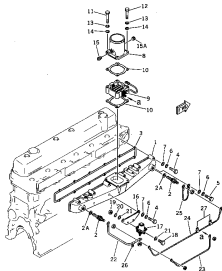
エアークレックマニホールドおよび コネクション 適用 号 機 FIG. 111 AIR INTAKE MANIFOLD AND CONNECTION (ENGINE NO. 16877 - 19206)
