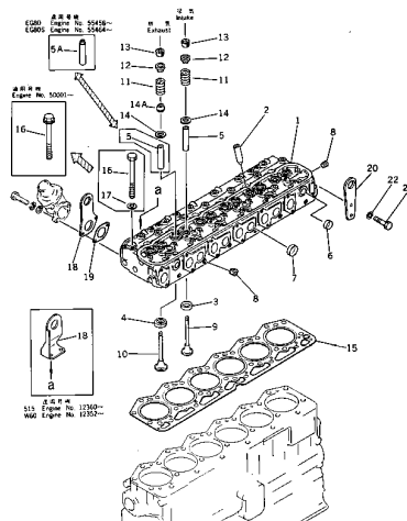
シリンダヘッド FIG. 101 CYLINDER HEAD
