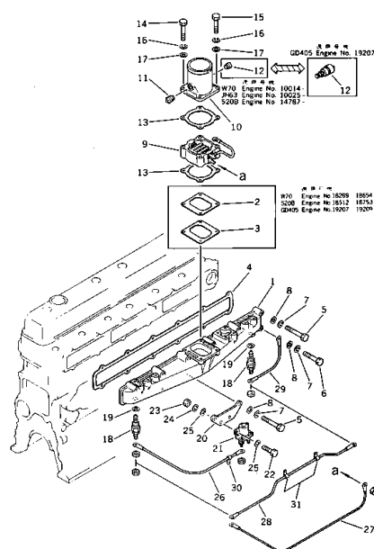
エア インテーク マニホールド および コネクション FIG. 111A AIR INTAKE MANIFOLD AND CONNECTION 適用機 (ENGINE NO.18450-)
