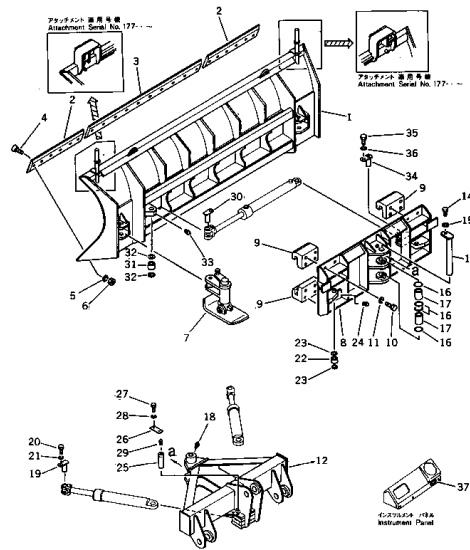
サイドシフト特、ピッチ、アングル スノー ブラウ Fig. 121 SIDE SHIFT, PITCH & ANGLE SNOW PLOW
