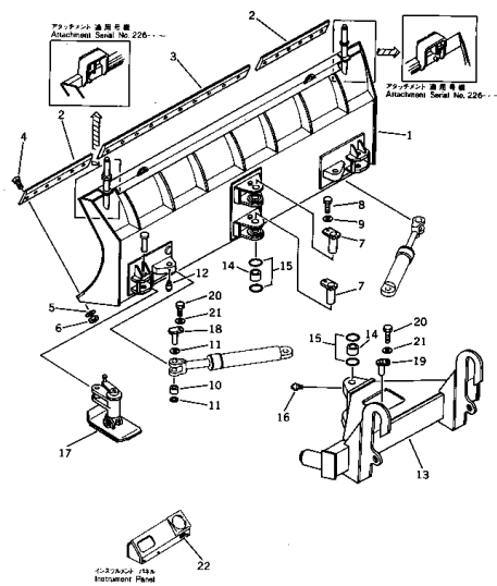
マルチカブラ用ピッチ式アングルスノーブロー Fig. 131 PITCH & ANGLE SNOW PLOW FOR MULTI COUPLER
