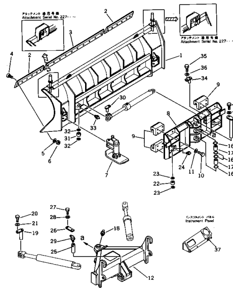
マルチコブラ用サイドシフトピッチ式 Fig. 141 SIDE SHIFT, PITCH & ANGLE SNOW PLOW アングルスノーブロー FOR MULTI COUPLER
