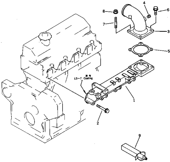
エアークリーナー マニホールド コネクション FIG. 1301 AIR INTAKE MANIFOLD CONNECTION 適用台数 (ENGINE NO. 10001 - 30835)
