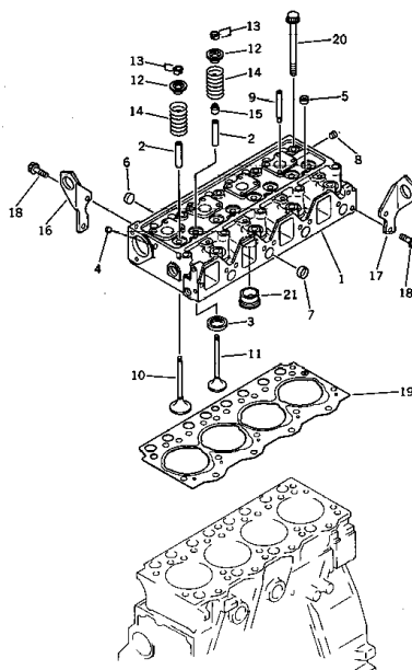
FIG. 1001 シリンダヘッド CYLINDER HEAD
