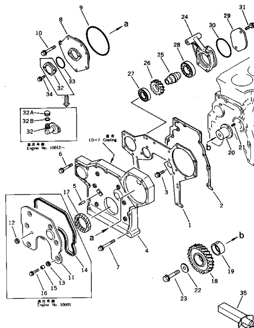
フロント カバー および ギヤー 適用 番 號 FIG. 2021 FRONT COVER AND GEAR (ENGINE NO. 10001 - 10024)
