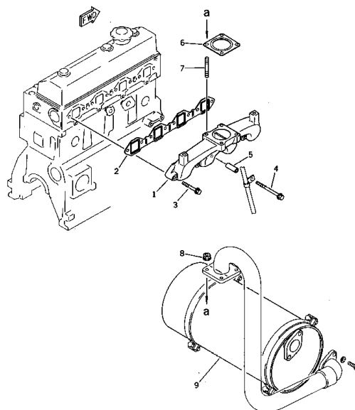
エキゾーストマニホールドおよびマフラー FIG. 1501 EXHAUST MANIFOLD AND MUFFLER
