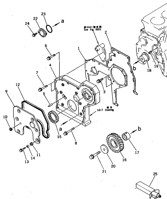
フロントカバー およびギヤー FIG. 2021 FRONT COVER AND GEAR
