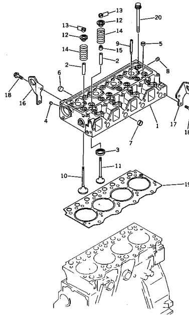
FIG. 1001 シリンダヘッド CYLINDER HEAD
