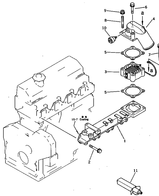
エアインテークマニホールドおよびコネクション FIG. 1301 AIR INTAKE MANIFOLD AND CONNECTION
