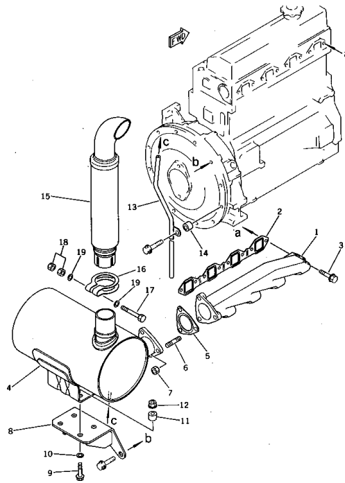
エキゾースト マニホールドおよびマフラー FIG. 1501 EXHAUST MANIFOLD AND MUFFLER
