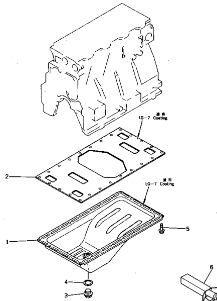
FIG. 2101 OIL PAN オイルパン
