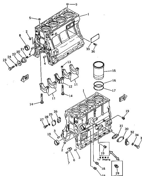
シリンダ ブロック Fig. 201 CYLINDER BLOCK
