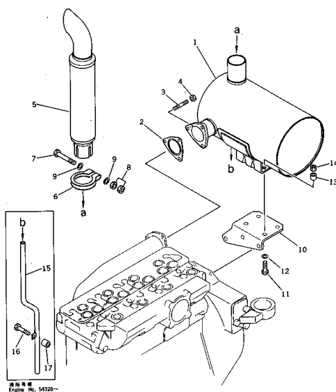
Fig. 181 マフラー MUFFLER
