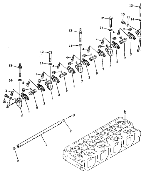
Fig. 103 ROCKER ARM
