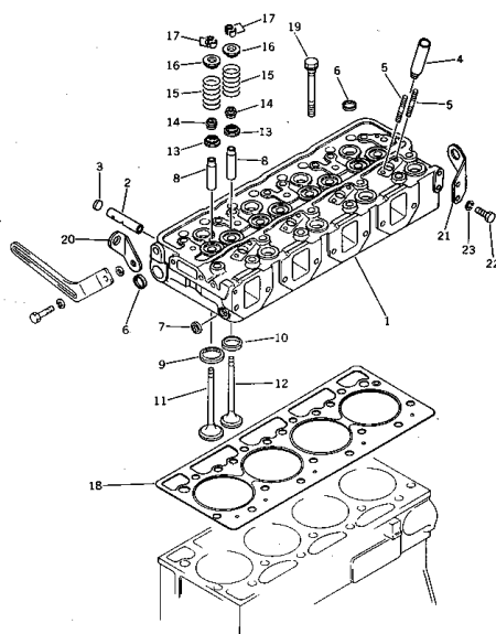
Fig. 101 シリンダヘッド CYLINDER HEAD
