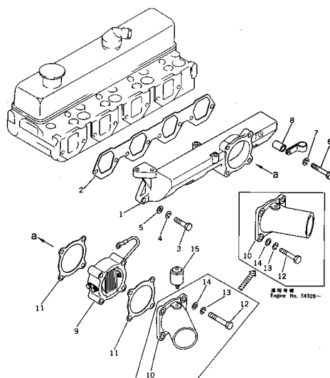
エアインテークマニホールド Fig. 111 AIR INTAKE MANIFOLD
