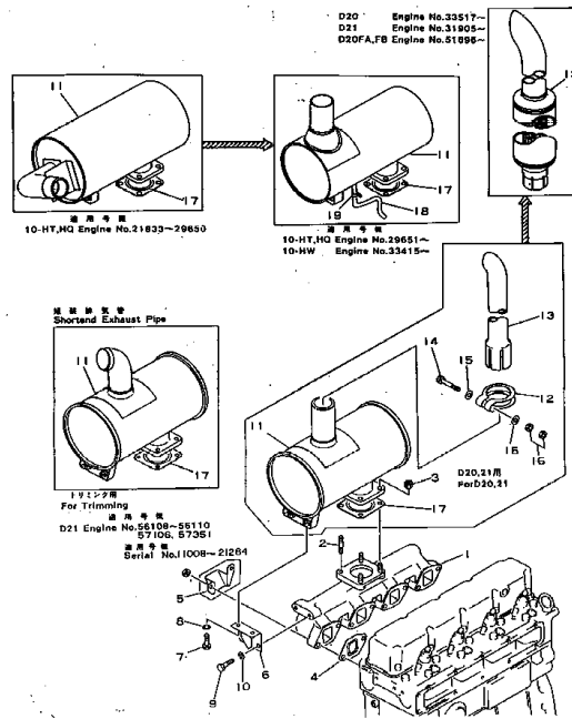
エキゾースト マニホールド および マフラー FIG. 121 EXHAUST MANIFOLD AND MUFFLER
