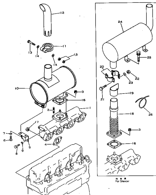
エキゾースト マニホールド および マフラー FIG. 124 EXHAUST MANIFOLD AND MUFFLER
