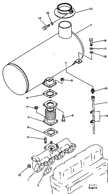
エキゾースト マニホールド および マ フ ラ 適用号機 FIG. 123 EXHAUST MANIFOLD AND MUFFLER (4D92-1F ENGINE NO. 41872 - )
