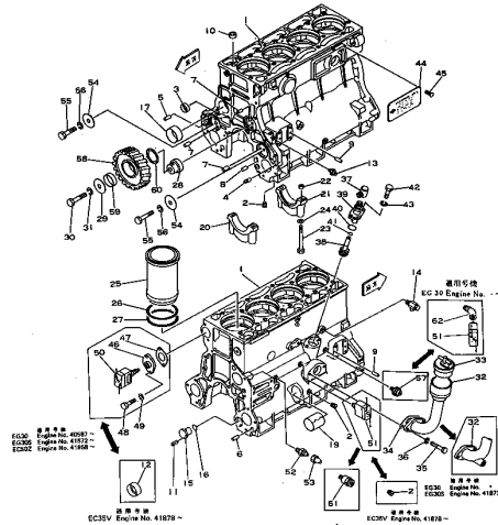
シリンドラ ブロック CYLINDER BLOCK
