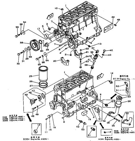
FIG. 202 CYLINDER BLOCK シリンダーブロック
