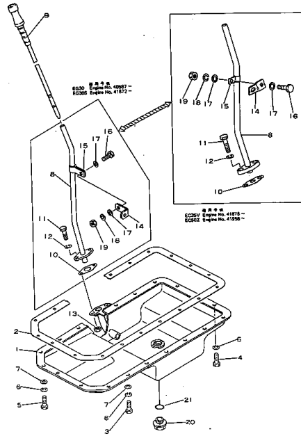
オイルパン FIG. 216 OIL PAN
