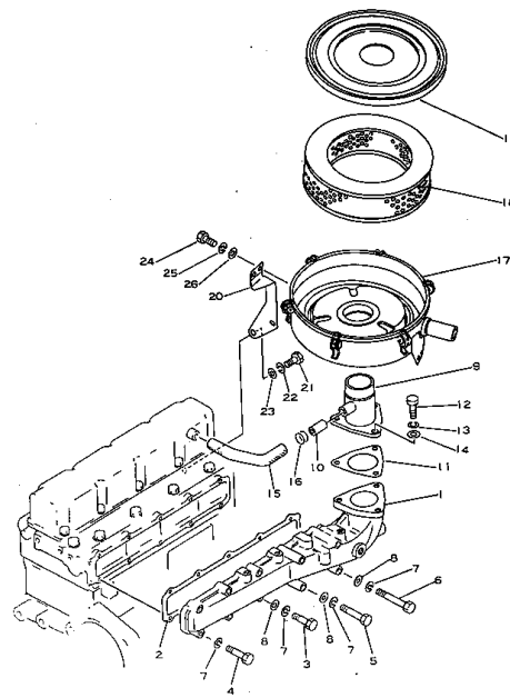
エア- インテーク マニホールド および エア- クリーナ 適用 号機 FIG. 113 AIR INTAKE MANIFOLD AND AIR CLEANER (4D92-1E ENGINE NO. 40587 - )
