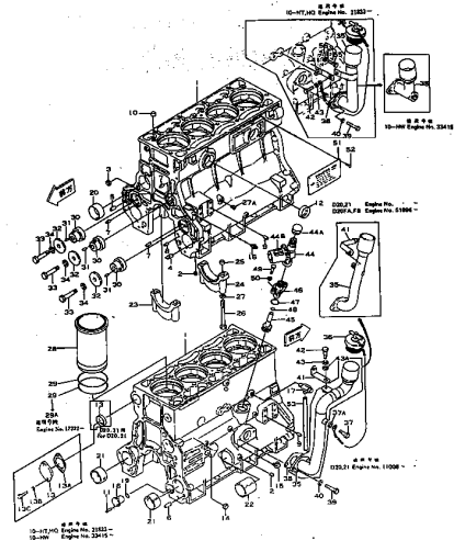
シリンダブロック CYLINDER BLOCK
