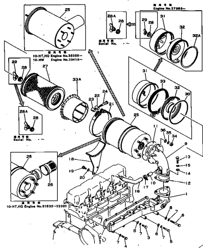
エア・インテークマニホールドおよびエアークリーナ FIG. 112 AIR INTAKE MANIFOLD AND AIR CLEANER
