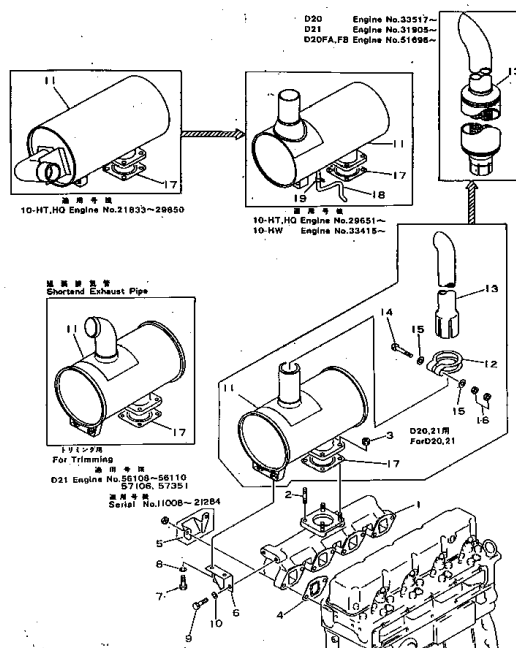
エキゾースト マニホールドおよび マ フ ラ FIG. 121 EXHAUST MANIFOLD AND MUFFLER
