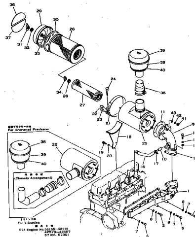
エアーインテークマニホールドおよびエアークリーナ FIG. 111 AIR INTAKE MANIFOLD AND AIR CLEANER
