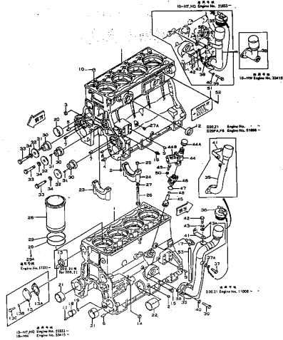
シリンダブロック FIG. 201 CYLINDER BLOCK
