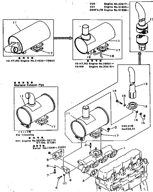
エキゾースト マニホールド および マフラー FIG. 121 EXHAUST MANIFOLD AND MUFFLER
