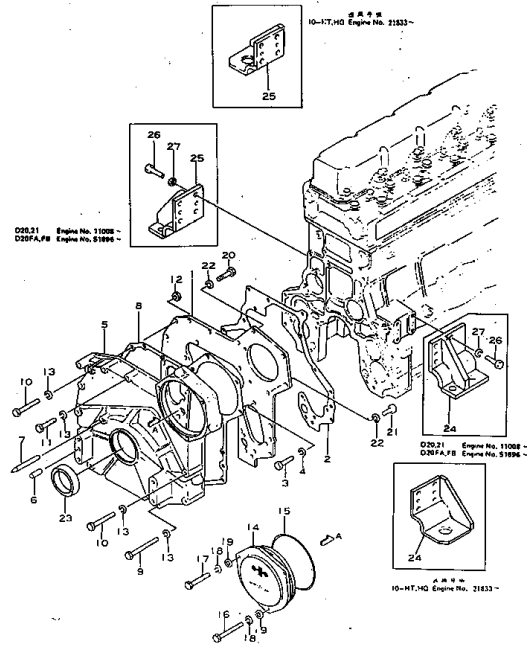
フロントカバー および プレート FIG. 211 FRONT COVER AND PLATE
