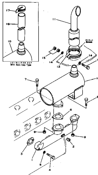
エキゾースト マニホールド および マフラー FIG. 121 EXHAUST MANIFOLD AND MUFFLER
