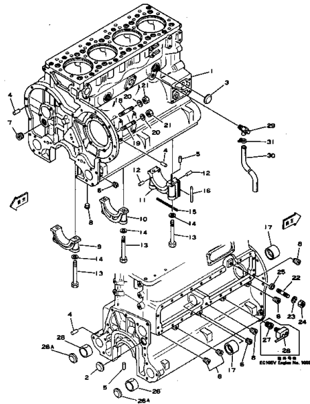
シリンダブロック FIG. 201 CYLINDER BLOCK (1/2)
