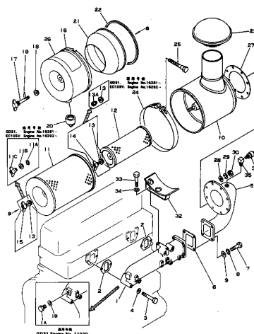
エアークリーナ マニホールドおよびエアークリーナ FIG. 111 AIR INTAKE MANIFOLD AND AIR CLEANER
