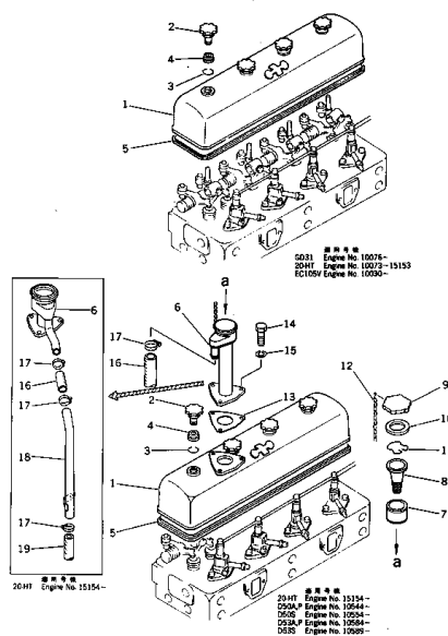
シリンダ ヘッド カバー FIG. 105 CYLINDER HEAD COVER
