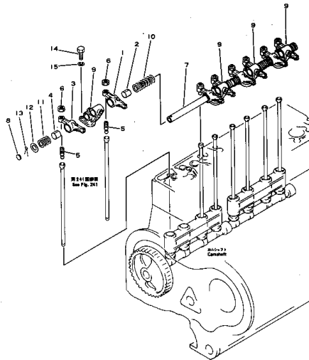
FIG. 103 ロッキングアーム ROCKER ARM
