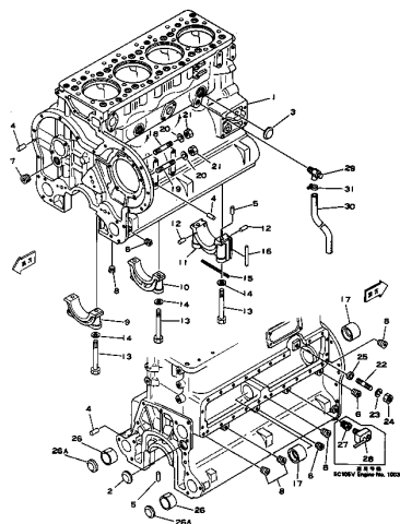
シリンダブロック FIG. 201 CYLINDER BLOCK (1/2)
