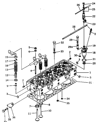
シリンダヘッド FIG. 101 CYLINDER HEAD
