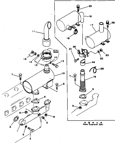
エキゾースト マニホールド および マフラー FIG. 123 EXHAUST MANIFOLD AND MUFFLER
