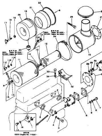
エアークリーナ マニホールドおよびエアークリーナ FIG. 111 AIR INTAKE MANIFOLD AND AIR CLEANER
