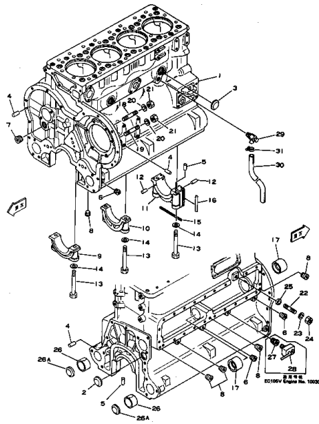
シリンダブロック FIG. 201 CYLINDER BLOCK (1/2)
