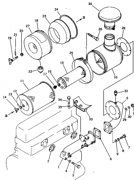
エア- インテーク マニホールド および エア- クリーナ Fig. 114 AIR INTAKE MANIFOLD AND AIR CLEANER (適用 機種 番号) (D53S-17 Engine No. 28323~)
