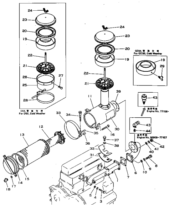
エアークリーナ マニホールド および エアークリーナ FIG. 1112 AIR INTAKE MANIFOLD AND AIR CLEANER 適用車種 (4D120-11B ENGINE NO. 89377-)
