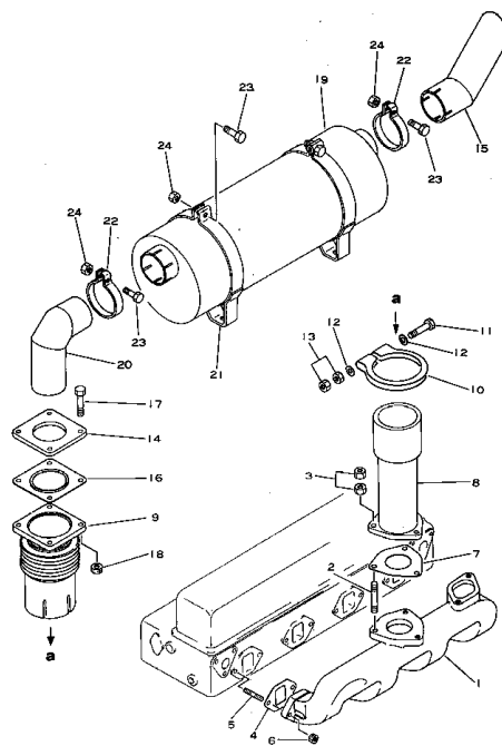
エキゾースト マニホールド および マフラー FIG. 1122 EXHAUST MANIFOLD AND MUFFLER (4D120-11B ENGINE NO. 89377- )
