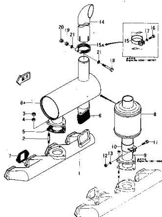
Fig. 102 エキゾースト マニホールド (適用 号 機 EXHAUST MANIFOLD (Engine No. 1301~49999))
