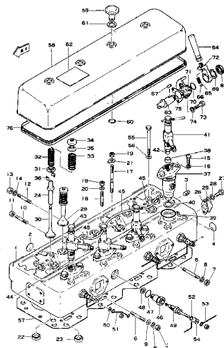
Fig. 101A シリンダヘッド、プリコンバッションチャンバ CYLINDER HEAD, PRECOMBUSTION CHAMBER およびコンプレッションリリース機構 (Engine No. 30255~49999)
