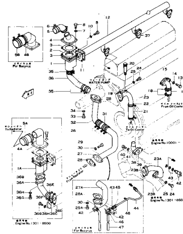
ウォーター マニホールド および サーモスタット ハウジング Fig. 103 WATER MANIFOLD AND THERMOSTAT HOUSING (適用車 Engine No. 1301~49999)
