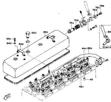
Fig. 101A シリンダヘッド、プリコンバッションチャンバ CYLINDER HEAD, PRECOMBUSTION CHAMBER ※207 コンプレッションリリース (適用機種) AND COMPRESSION RELEASE (2/2) (Engine No. 1301~30254)
