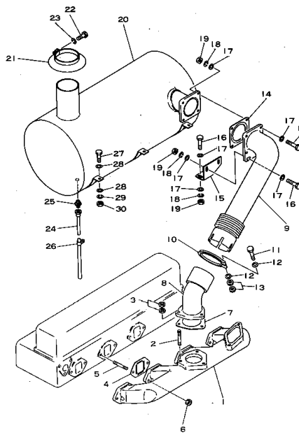
エキゾースト マニホルド および マフラー 適用機種 FIG. 1123 EXHAUST MANIFOLD AND MUFFLER (4D120-11D ENGINE NO. 89959 - )
