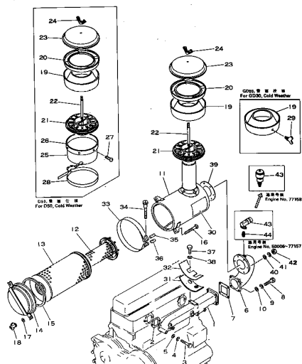
FIG. 1112 エアークリーナとエアークリーナホルダの分解図 FIG. 1112 AIR INTAKE MANIFOLD AND AIR CLEANER
