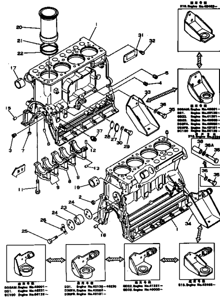
シリンダブロック FIG. 1201 CYLINDER BLOCK
