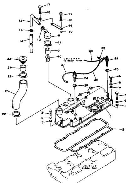
シリンダヘッドカバー 爆発図 FIG. 1105A CYLINDER HEAD COVER (ENGINE NO.63877-)
