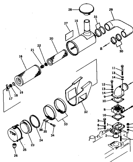
エアークリーナコネクショおよびエアークリーナ FIG. 1111A AIR INTAKE CONNECTION AND AIR CLEANER 適用機種 (ENGINE NO.63877-)
