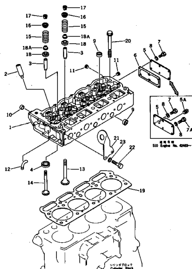
シリンダヘッド FIG. 1101 CYLINDER HEAD
