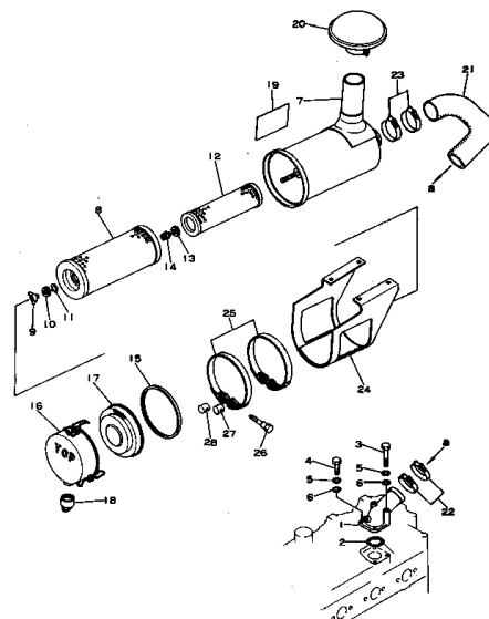
エアークリーナ コネクション および エアークリーナ FIG. 1111 AIR INTAKE CONNECTION AND AIR CLEANER 適用 機種 (ENGINE NO.57899-63876)
