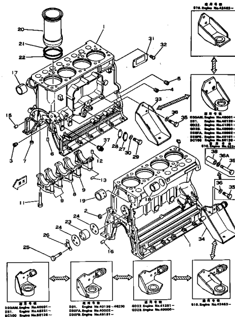
FIG. 1201 シリンダ ブロック CYLINDER BLOCK
