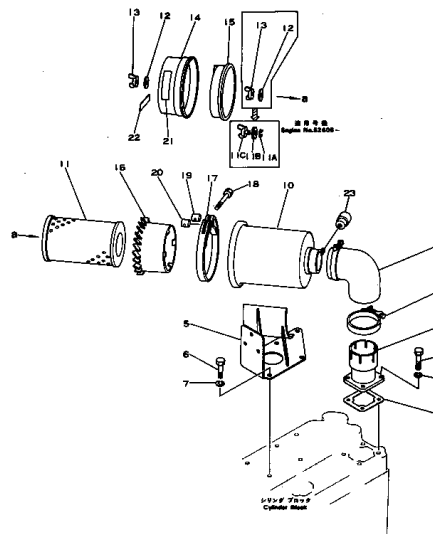
エアー インテーク コネクション および エアー クリーナ FIG. 114 AIR INTAKE CONNECTION AND AIR CLEANER 適用 機種 (EG45 ENGINE NO. 30066- )
