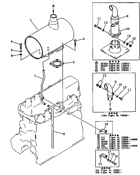
マフラー FIG. 2181 MUFFLER
