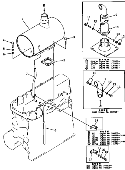
マフラー FIG. 2181 MUFFLER
