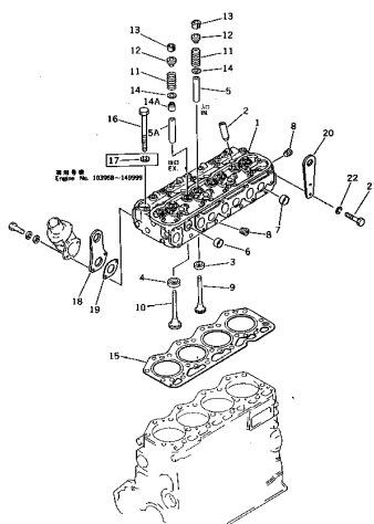
FIG. 2102 シリンダヘッド FIG. 2102 CYLINDER HEAD
