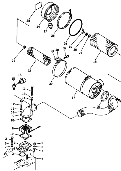
エアークリーナコネクショ、リボンヒータおよびエアークリーナ FIG. 1116 AIR INTAKE CONNECTION, RIBBON HEATER AND AIR CLEANER
