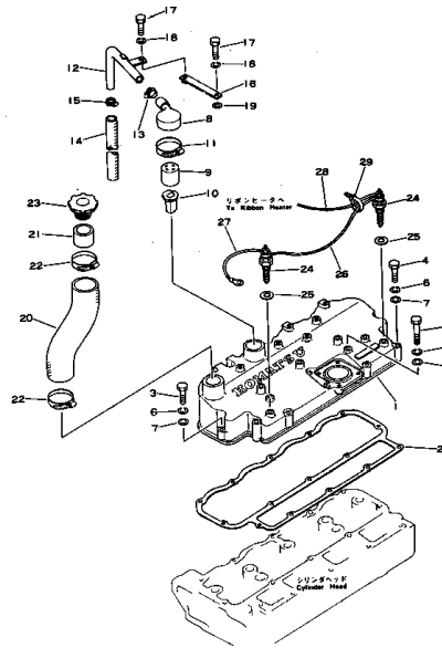
シリンダヘッドカバー FIG. 1105 CYLINDER HEAD COVER
