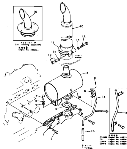
エキゾーストマニホールドおよびマフラー FIG. 1121 EXHAUST MANIFOLD AND MUFFLER
