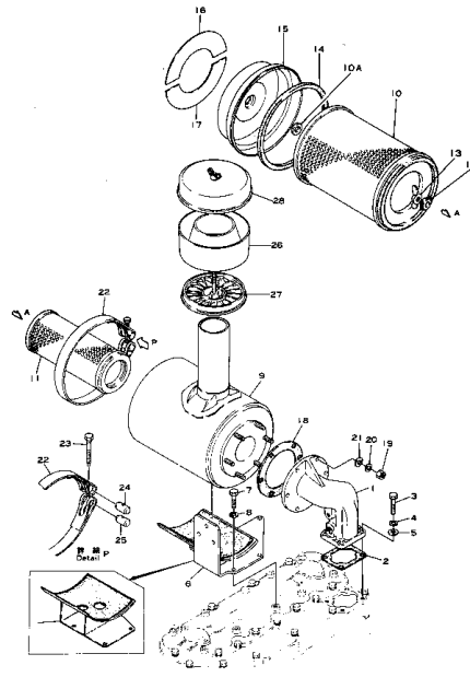
エアークリーナ接続およびエアークリーナ FIG. 113 AIR INTAKE CONNECTION AND AIR CLEANER
