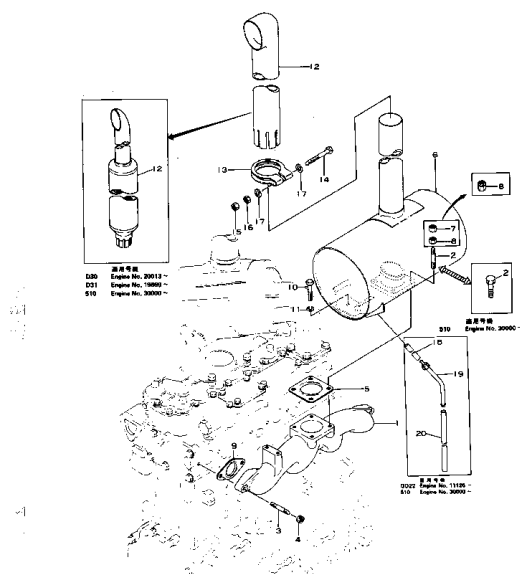
エキゾーストマニホールドおよびマフラー FIG. 121 EXHAUST MANIFOLD AND MUFFLER
