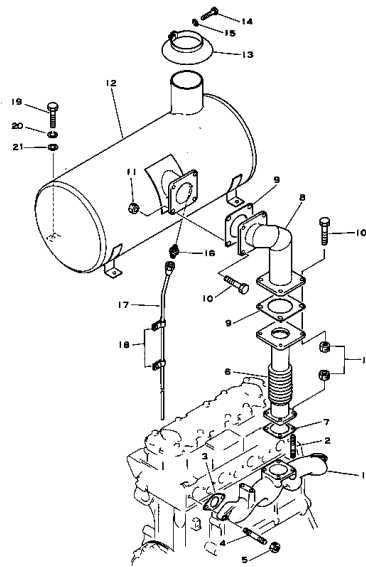
エキゾースト マニホールド および マフラー 適用 参考 FIG. 123 EXHAUST MANIFOLD AND MUFFLER (EG45S ENGINE NO. 30083- )
