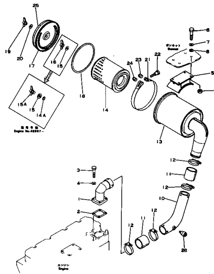
エアー インテーク コネクション および エアー クリーナ FIG. 115 AIR INTAKE CONNECTION AND AIR CLEANER 適用機種 (EG45S ENGINE NO. 30083-)
