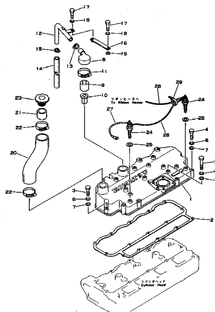
シリンダヘッドカバー 通用号機 FIG. 1105A CYLINDER HEAD COVER (ENGINE NO. 63806 -)
