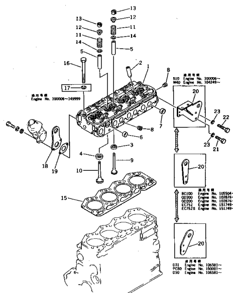
シリンダヘッド FIG. 2101 CYLINDER HEAD
