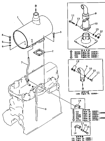
マフラー FIG. 2181 MUFFLER
