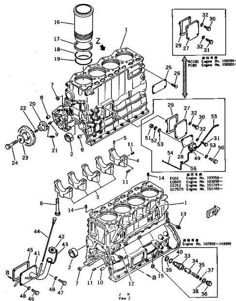
シリンダブロック FIG. 2202 CYLINDER BLOCK
