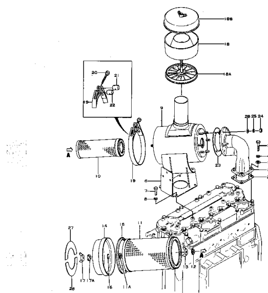
エアインテーク コネクション および エアークリーナ FIG. 111 AIR INTAKE CONNECTION AND AIR CLEANER
