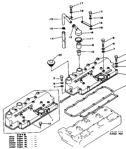
シリンダヘッドカバー FIG. 1106 CYLINDER HEAD COVER
