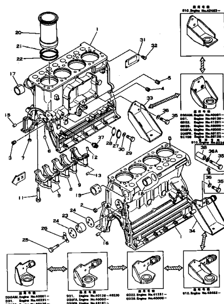
シリンダブロック FIG. 1201 CYLINDER BLOCK
