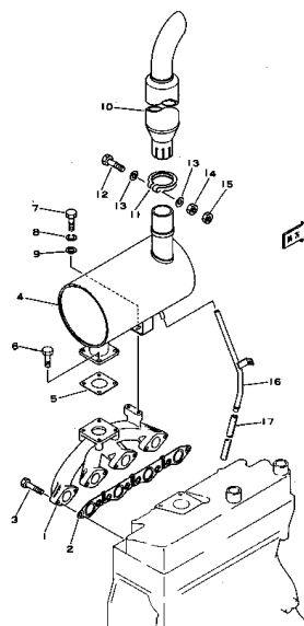
エキゾーストマニホールドおよびマフラー FIG. 1123 EXHAUST MANIFOLD AND MUFFLER
