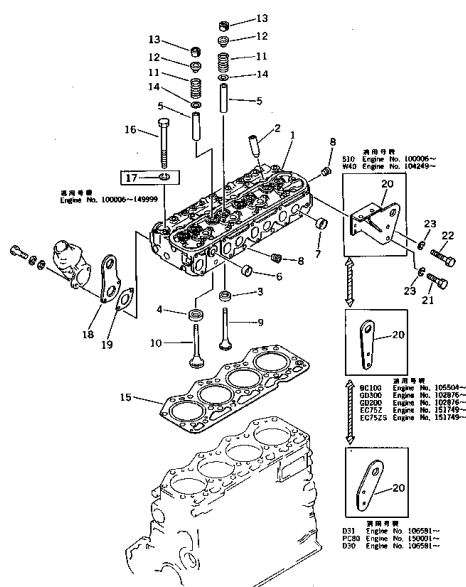
FIG.2101 シリンダ ヘッド CYLINDER HEAD
