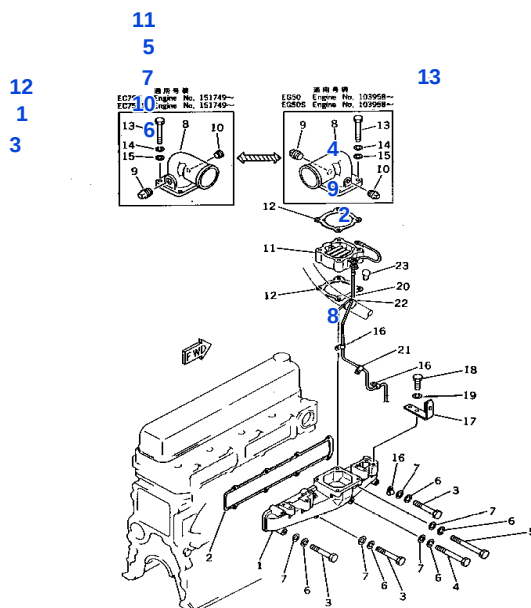
エアー インテーク マニホールド および コネクション FIG. 2112 AIR INTAKE MANIFOLD AND CONNECTION
