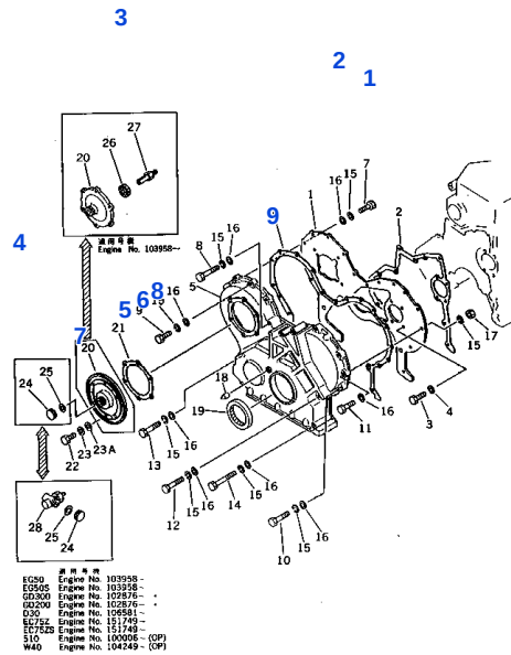
FIG. 2211 フロアカバー FRC COVER
