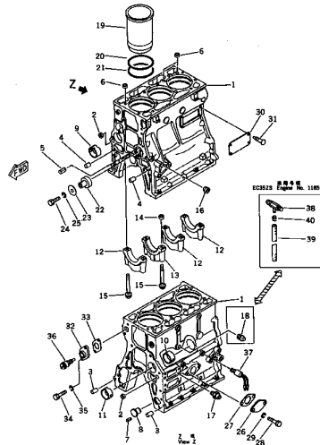
シリンダ ブロック FIG. 202 CYLINDER BLOCK
