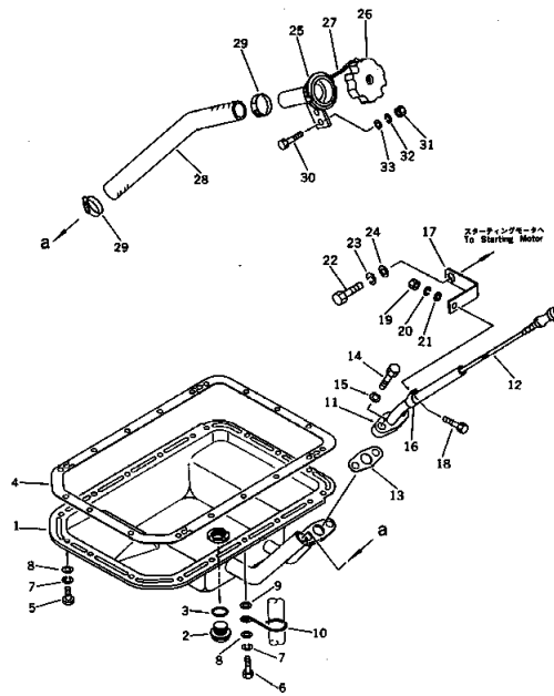
オイル パン 適用機種 FIG. 216 OIL PAN (EC36Z ENGINE NO. 11852-)
