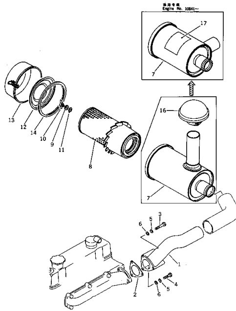
エアークリーナ FIG. 161 AIR CLEANER
