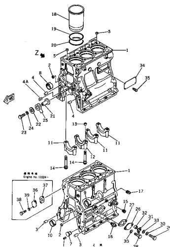
シリンダブロック FIG. 201 CYLINDER BLOCK
