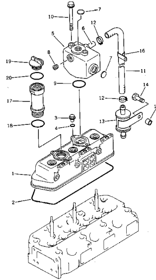
シリンダヘッドカバー 適用機種 FIG. 107 CYLINDER HEAD COVER (ENGINE NO.05810- )
