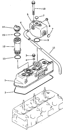
シリンダヘッドカバー 適用機種 FIG. 106A CYLINDER HEAD COVER (ENGINE NO.05590-05809)
