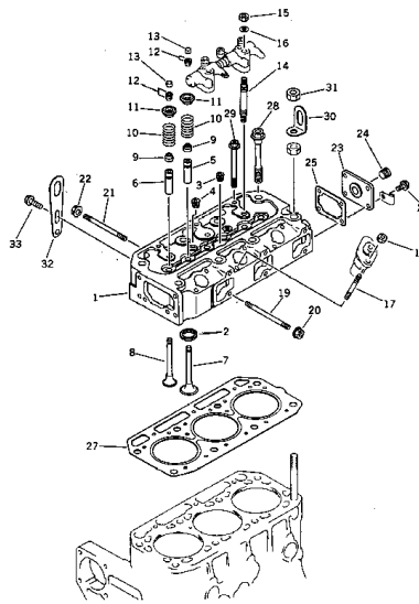
シリンダヘッド FIG. 102 CYLINDER HEAD
