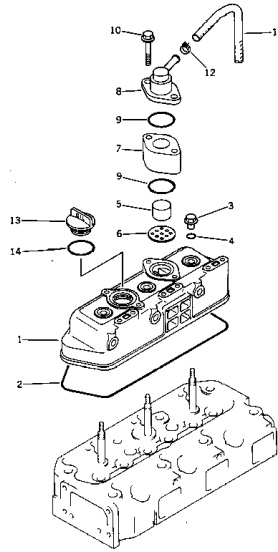
シリンダヘッドカバー 適用機種 FIG. 106 CYLINDER HEAD COVER (ENGINE NO.01001-05589)
