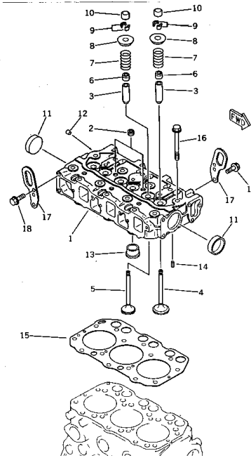
シリンダ ヘッド FIG. 1001 CYLINDER HEAD
