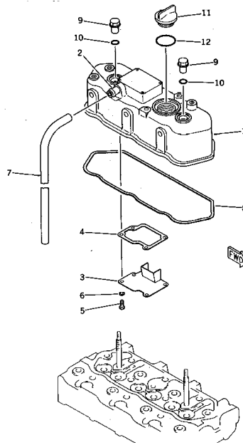
シリンダ ヘッド カバー FIG. 1151 CYLINDER HEAD COVER
