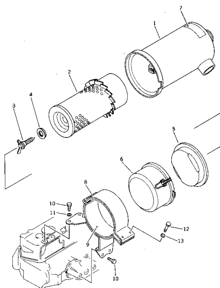
Fig. 161 エアークリーナ AIR CLEANER
