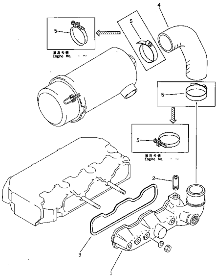
Fig. 111 エアー インテーク マニホールド AIR INTAKE MANIFOLD
