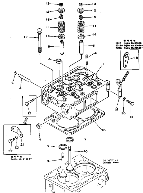
シリンダヘッド FIG. 1101 CYLINDER HEAD
