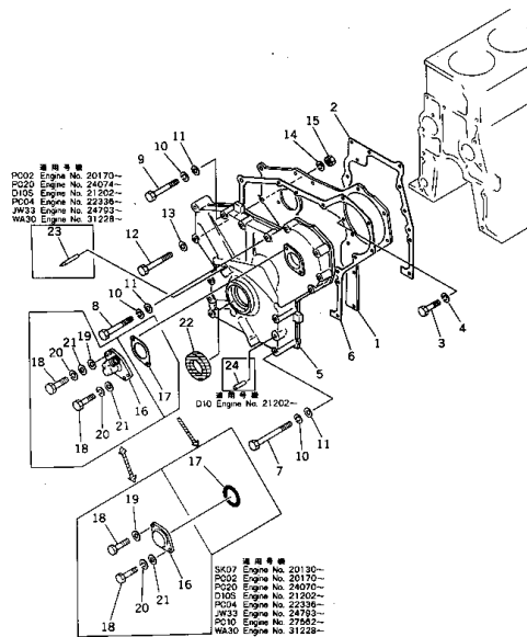
ギヤー カバー およびプレート FIG. 1211 GEAR COVER AND PLATE
