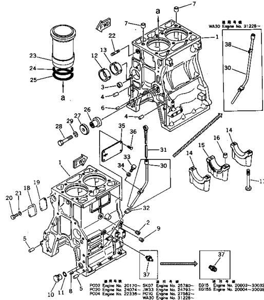
シリンダブロック FIG. 1201 CYLINDER BLOCK
