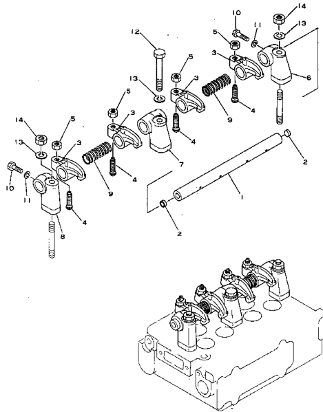
ロ ッ カ アーム FIG. 1103 ROCKER ARM
