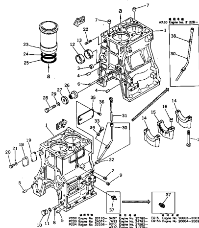
シリンダブロック FIG. 1201 CYLINDER BLOCK
