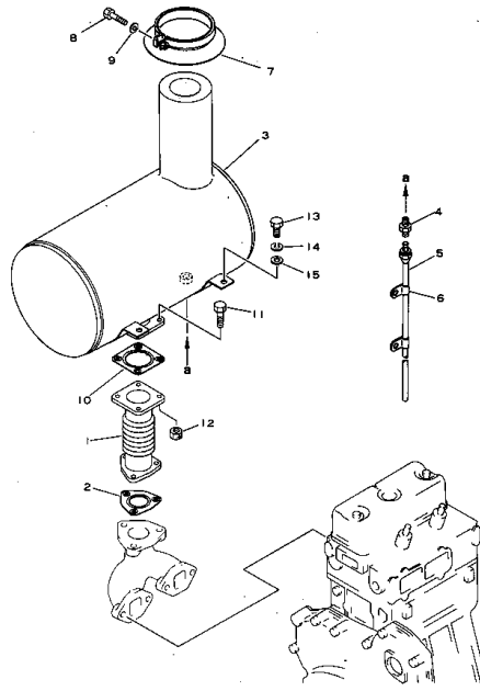
マフラー 適用機種 FIG. 1185 MUFFLER (EG15S ENGINE NO. 20004 - 30038)
