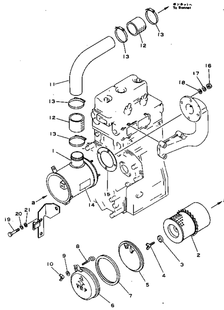
エアークリーナ 適用機種 FIG. 1164 AIR CLEANER (EG15S ENGINE NO. 20004 - 30038)
