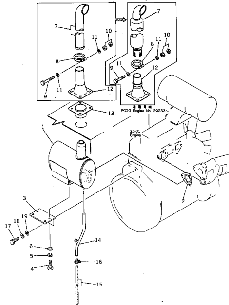
マフラー FIG. 1183 MUFFLER
