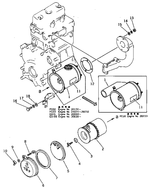
エアークリーナ FIG. 1163 AIR CLEANER
