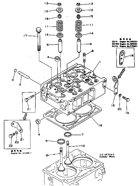
シリンダヘッド FIG. 1101 CYLINDER HEAD
