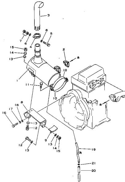
マフラー FIG. 1181 MUFFLER
